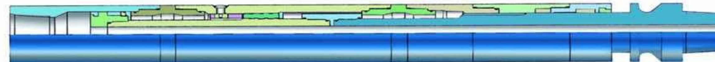
ZSJ/ZXJ型机械液压两体式震击器 ZSJ/ZXJ Hydraulic & Mechanical
